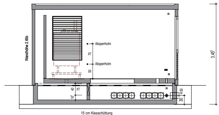
Längsschnitt
